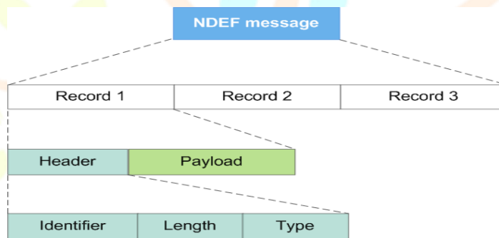
Fig. 6. NDEF message
