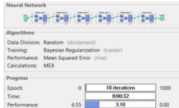
Fig.8 Deep Net Parameters
